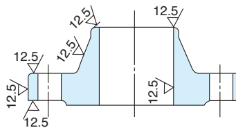
突合せ溶接式フランジ(WN)
