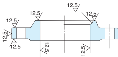
ハブフランジ(SOH) ハブフランジA形
